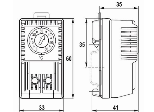
Рис. 1а – Общий вид и габаритные размеры термостатов UNISPLIT 35NCF02 и UNISPLIT 36NOF01
