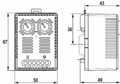
Рис. 1б – Общий вид и габаритные размеры термостата UNISPLIT 71NCNOF01
