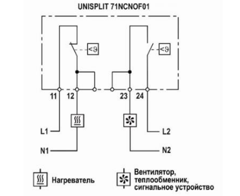
Рис. 2б - Электрическая схема подключения термостата UNISPLIT 71NCNOF01
