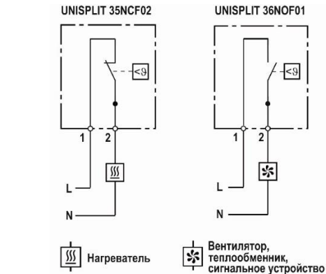
Рис. 2а - Электрические схемы подключения термостатов UNISPLIT 35NCF02 и UNISPLIT 36NOF01
